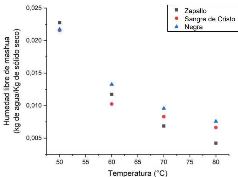
Figura 2. Efecto de la temperatura de secado en la humedad libre (kg de agua/kg de sólido seco) de la mashua zapallo, sangre de Cristo y negra.
