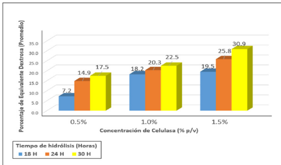
Figura 4. Relación entre la concentración de la enzima celulasa y el tiempo de hidrólisis con el porcentaje de equivalente de dextrosa
