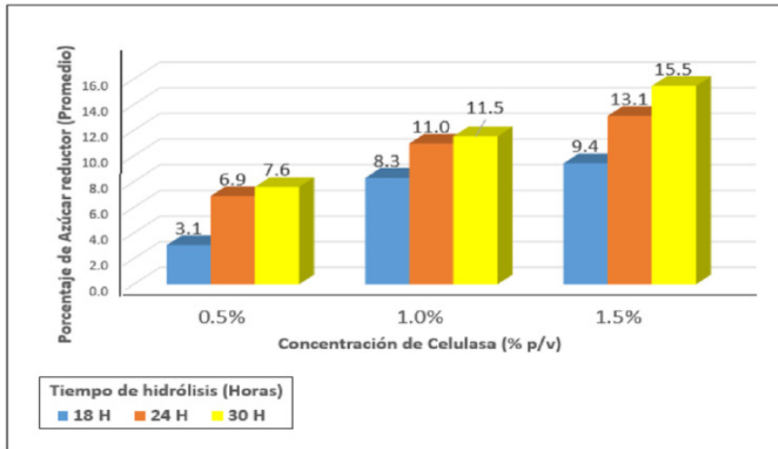
Figura 3. Relación entre la concentración de la enzima celulasa y el tiempo de hidrólisis con el % azúcares reductores (AR)
