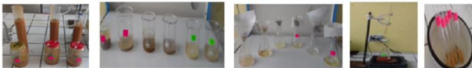
Figura 2. Fotografías del desarrollo del proceso de hidrólisis de cáscaras de plátano
