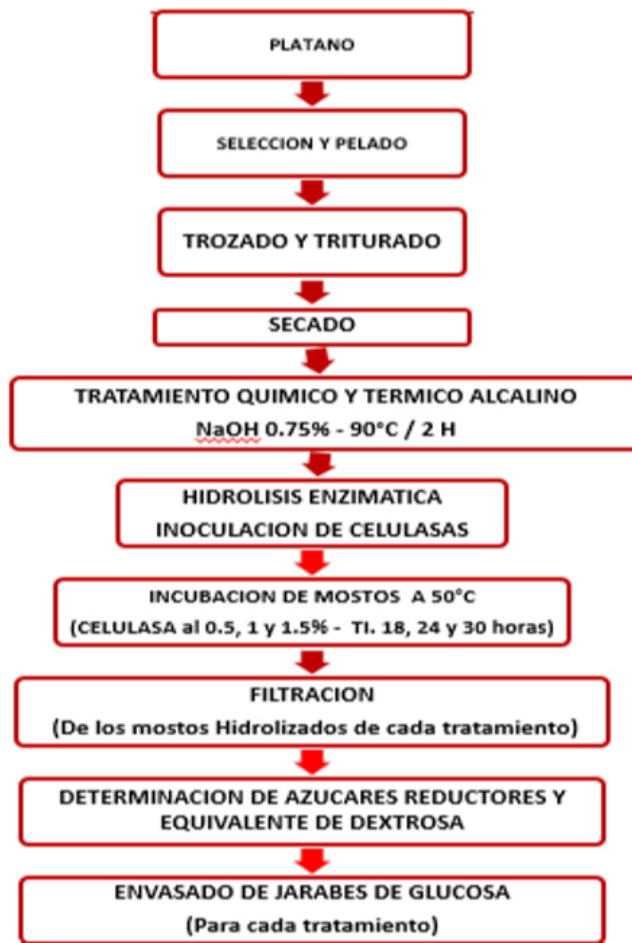
Figura 1. Diagrama del proceso de hidrólisis enzimática aplicado a las cáscaras de plátano
